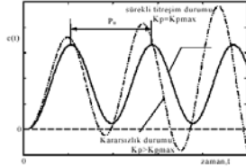
Şekil 7.12 Titreşim yöntemi
