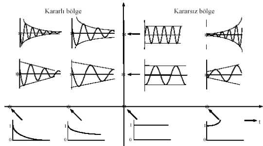
Şekil 6.2 Köklerin s-düzlemindeki yerlerine bağlı olarak değişen çeşitli anidarbe cevap eğrileri
